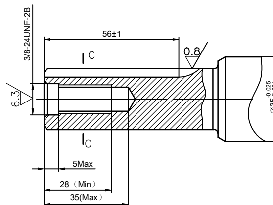
曲轴输出端接口尺寸
