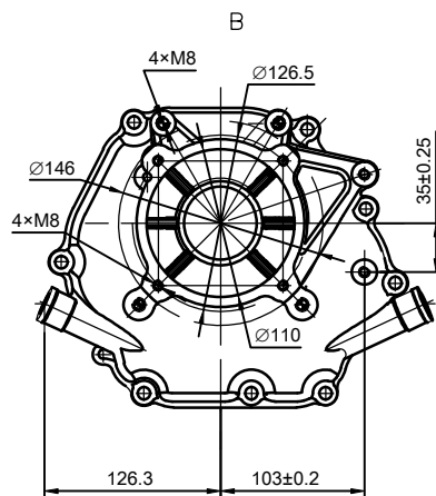
箱盖接口尺寸
